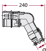
Fiche / Plug 50°
