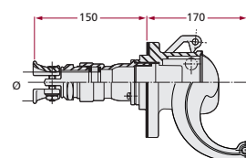
Boîtier coupleur Coupling socket
